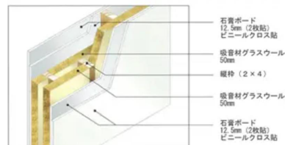
界壁断面図（1時間準耐火構造）
