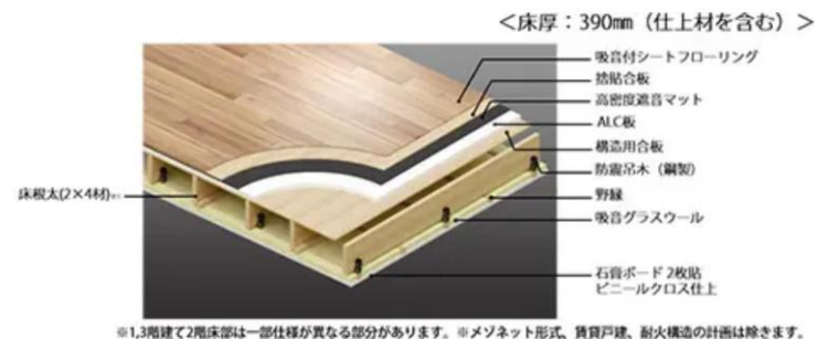
界床断面図（1時間準耐火構造）
